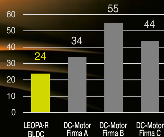
Messergebnisse der Temperatur von Kaltluft (°C)
