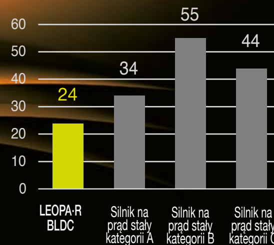
Wyniki pomiarów temperatury zimnego powietrza (°C)
